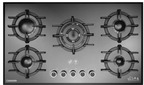
G639 Glass Gas Hobs Dimensions: 52x88 cm Cutting dimensions: 48x84 cm اجاق گاز رومیزی
